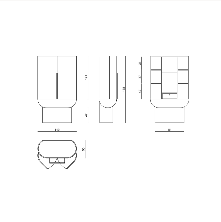
SIOSM3 L 110 x H 188 x W 50 cm
