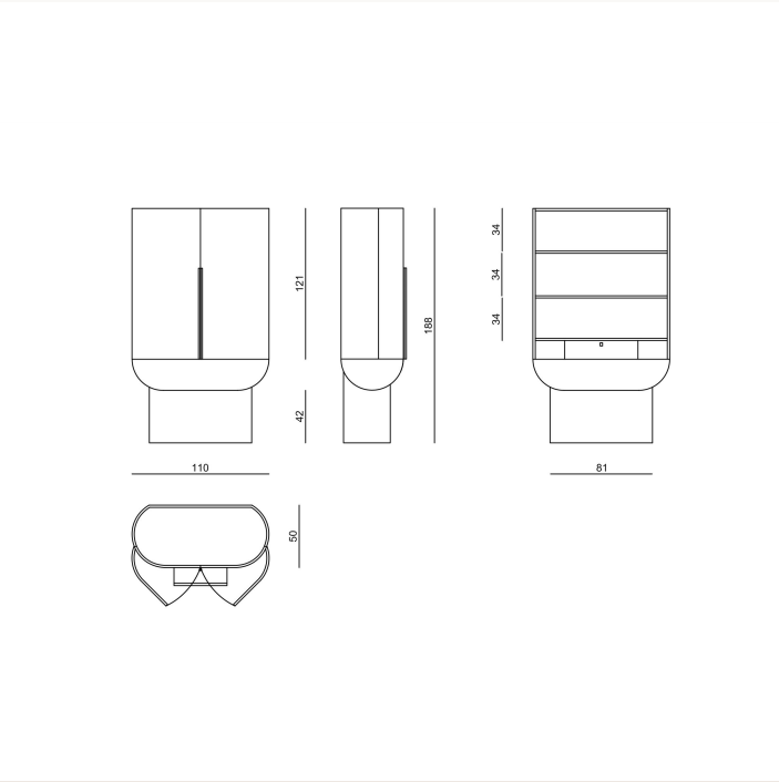
SIOSM2 L 110 x H 188 x W 50 cm
