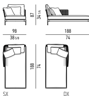
CHAISE-LONGUE CM 98X188 CHAISE-LONGUE CM 98X188
