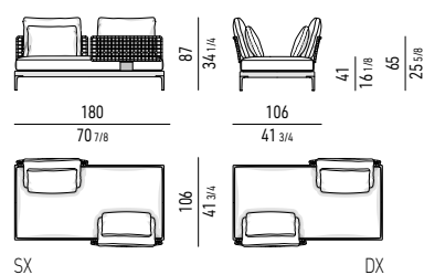
ELEMENTO CENTRALE VIS-À-VIS CM 180X106 VIS-À-VIS CENTRAL ELEMENT CM 180X106
