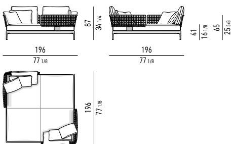
ISOLA VIS-À-VIS CM 196X196 VIS-À-VIS ISLAND CM 196X196
