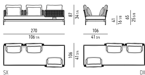
ELEMENTO CENTRALE VIS-À-VIS CM 270X106 VIS-À-VIS CENTRAL ELEMENT CM 270X106
