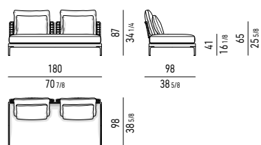
ELEMENTO CENTRALE CM 180X98 CENTRAL ELEMENT CM 180X98
