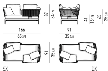
DIVANO VIS-À-VIS CM 166X91 VIS-À-VIS SOFA CM 166X91
