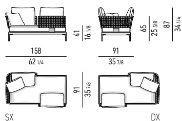
ELEMENTO TERMINALE VIS-À-VIS CM 158X91 VIS-À-VIS ELEMENT WITH 1 ARMREST CM 158X91
