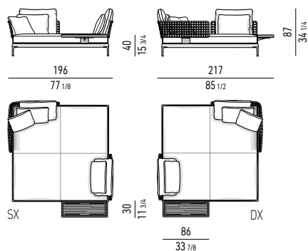
ISOLA VIS-À-VIS CON TOP CM 196X217 VIS-À-VIS ISLAND WITH TOP CM 196X217
