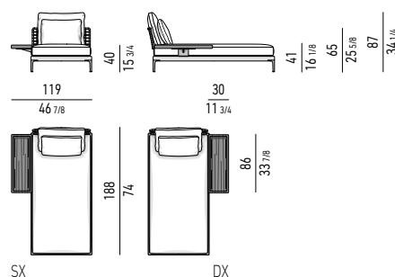
CHAISE-LONGUE CON TOP CM 119X188 CHAISE-LONGUE WITH TOP CM 119X188
