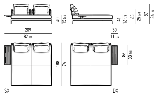
DOPPIO COUCH CON TOP CM 209X188 DOUBLE COUCH WITH TOP CM 209X188
