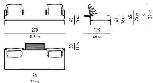
ELEMENTO CENTRALE OPEN CON TOP CM 270X119 OPEN CENTRAL ELEMENT WITH TOP CM 270X119
