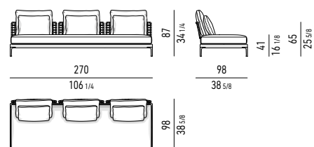
ELEMENTO CENTRALE CM 270X98 CENTRAL ELEMENT CM 270X98
